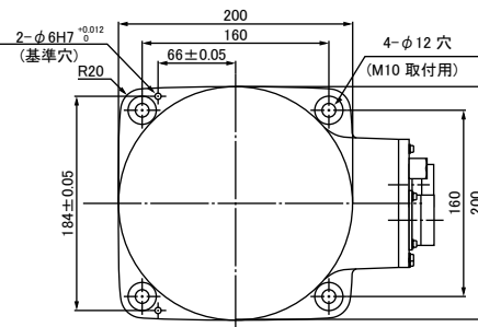
ベース取付面(上面より)
