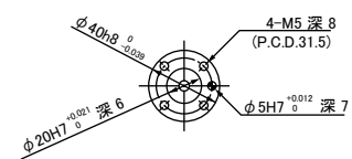
ベース取付面(上面より)
