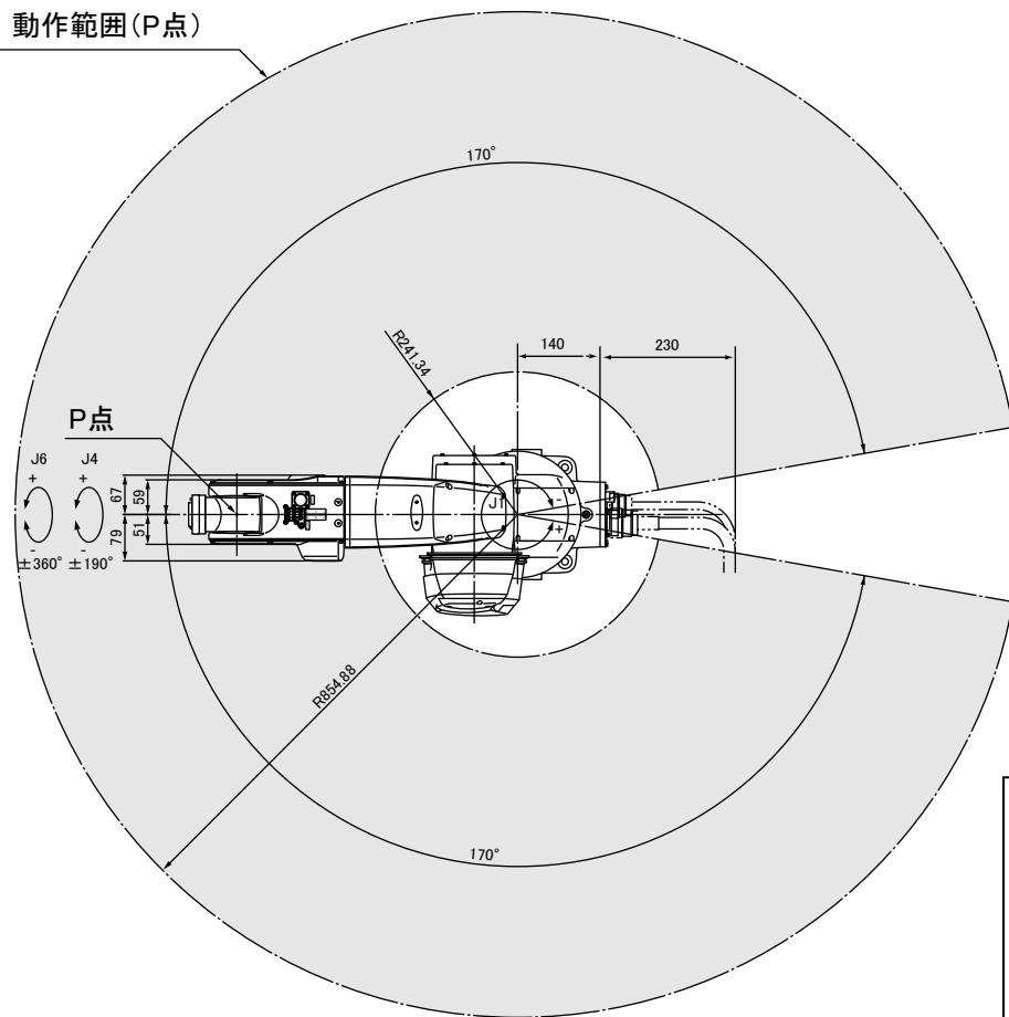
ツール取付面詳細(矢視A)
